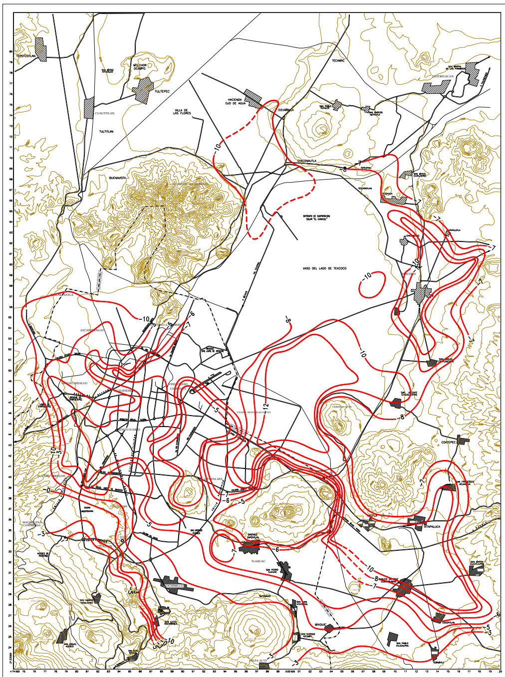
Figura 10. Evolución del nivel estático período 1996-2002
